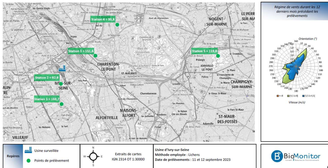
Carte des résultats en métaux en mg/kg de matière sèche dans les lichens observés lors de la campagne 2023
